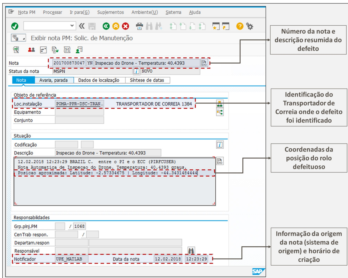
Figura 78 – Nota de Manutenção criada no CMMS com as informações enviadas pela UPE. Fonte: autor
