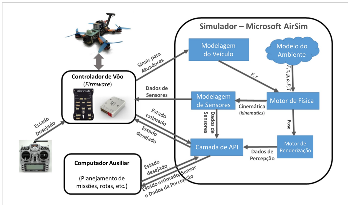
Figura 51 – Arquitetura do simulador Microsoft AirSim e interação com elementos externos. Fonte: traduzido de SHAH et al., 2017
