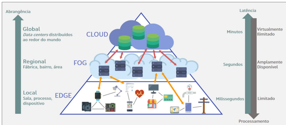
Figura 37 – Representação dos paradigmas de computação Edge , Fog e Cloud com sua respectiva abrangência. Fonte: adaptado de SPOTNITZ, 2017
