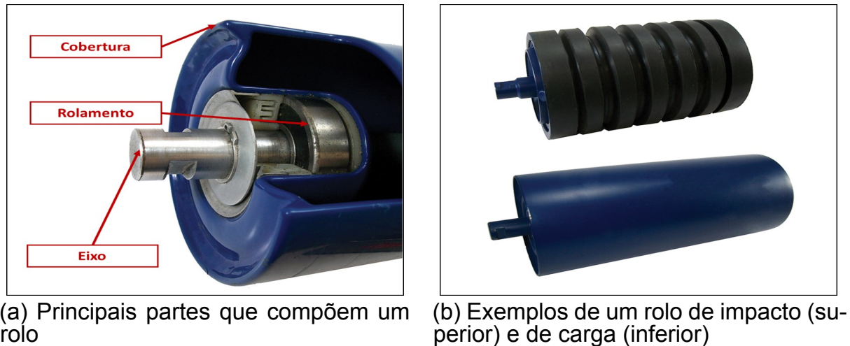
Figura 13 – Partes principais dos rolos e exemplos de alguns tipos de rolos. Fonte: adaptado de HCD CONVEYORS, 2017
